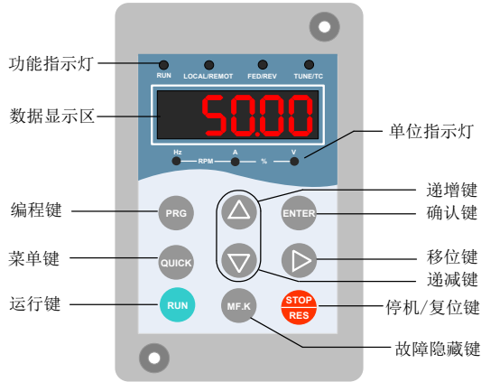
图 4-1 LED 操作面板
