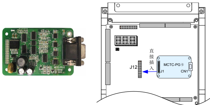
图 3-8 MCTC-PG 卡实物及安装示意图
