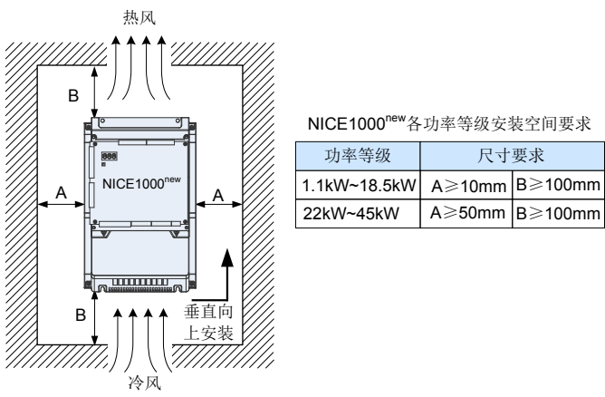
图 3-1 安装距离示意图
