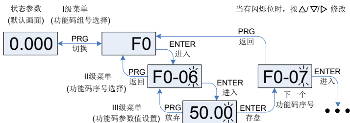
图 4-2 三级菜单操作流程图中
