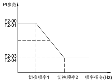
图 7-1 PI 参数示意图
