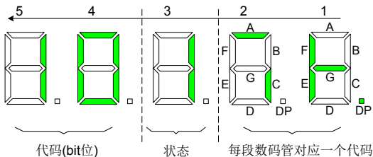
图 7-9 输入状态示例
