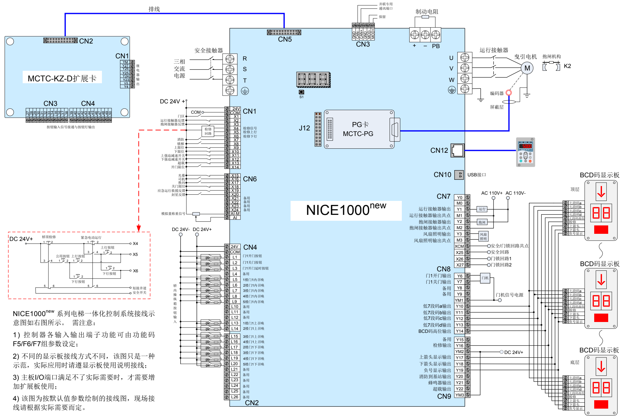
图 3-10 NICE1000 new 一体化控制系统接线示意图
