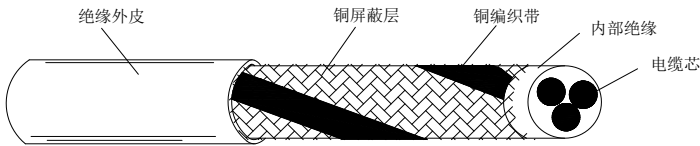
图 9-2 屏蔽层的编织密度要求
