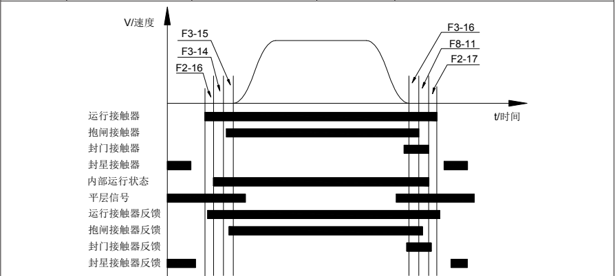
图 5-4 运行时序图
