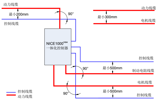
图 9-5 线缆布线要求
