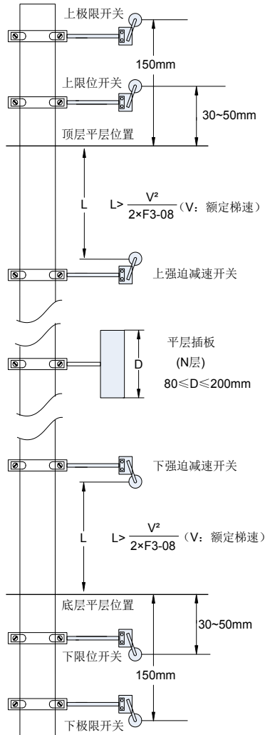
图 3-11 井道位置信号安装示意图
